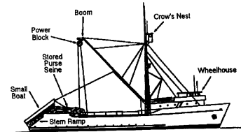
Purse Seiner
